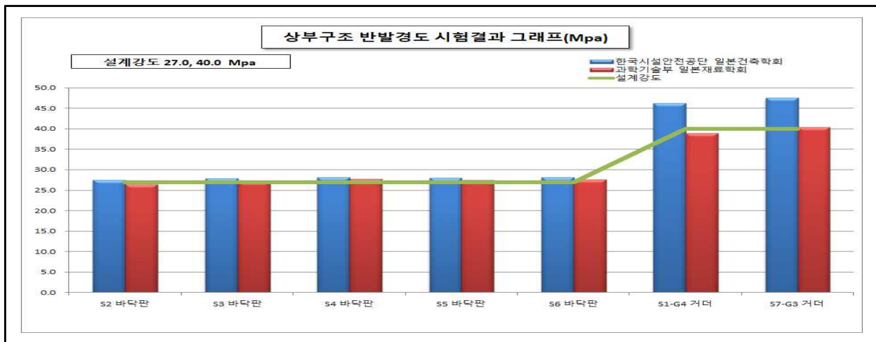
【그림 18.4.5】 영천방향 상부구조 반발경도시험 측정결과
