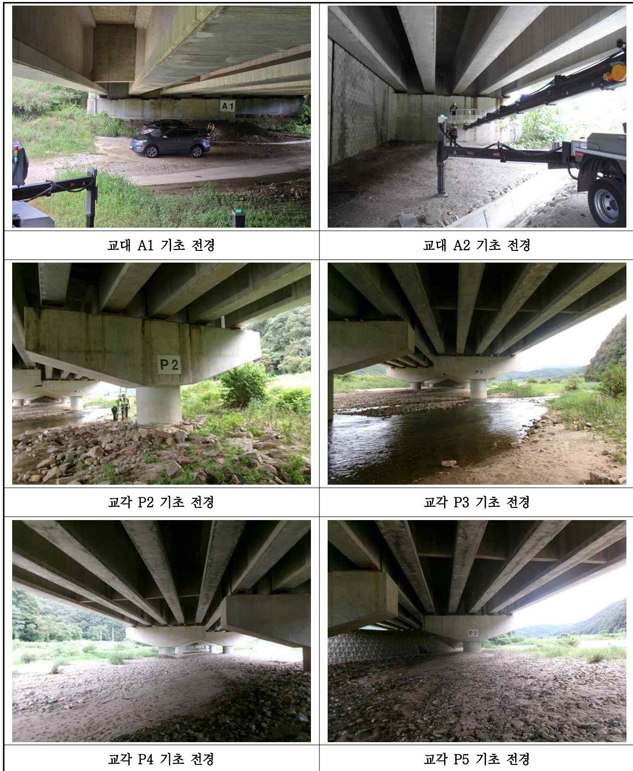
【사진 18.3.39】 기초 전경
